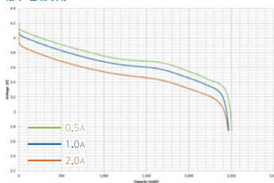
放電波形
