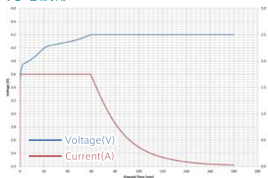
充電波形
