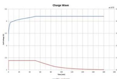
充電波形
